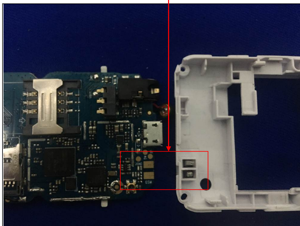
GSM Antenna
