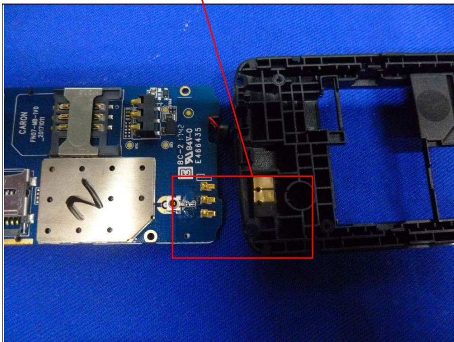
WWAN Antenna
