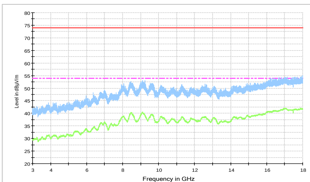
RE - 3GHz-18GHz
