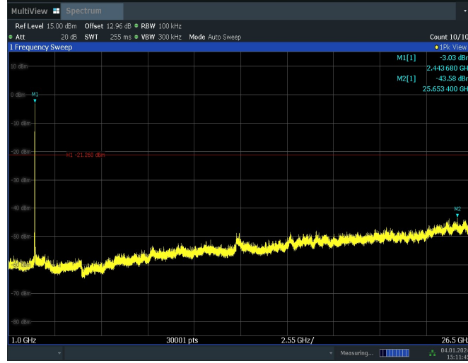
11AX20MIMO_Ant6_2437_52Tone_RU40_1000~26500
