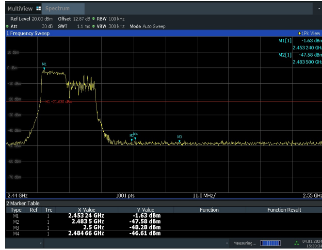
11AX20MIMO_Ant6_High_2462_106Tone_RU54
