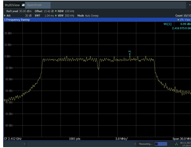
11N20MIMO_Ant10_2412_0~Reference
