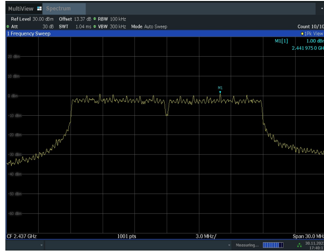
11N20MIMO_Ant10_2437_0~Reference
