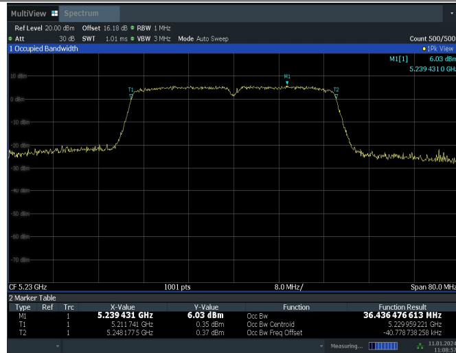
11N40MIMO_Ant6_5230
