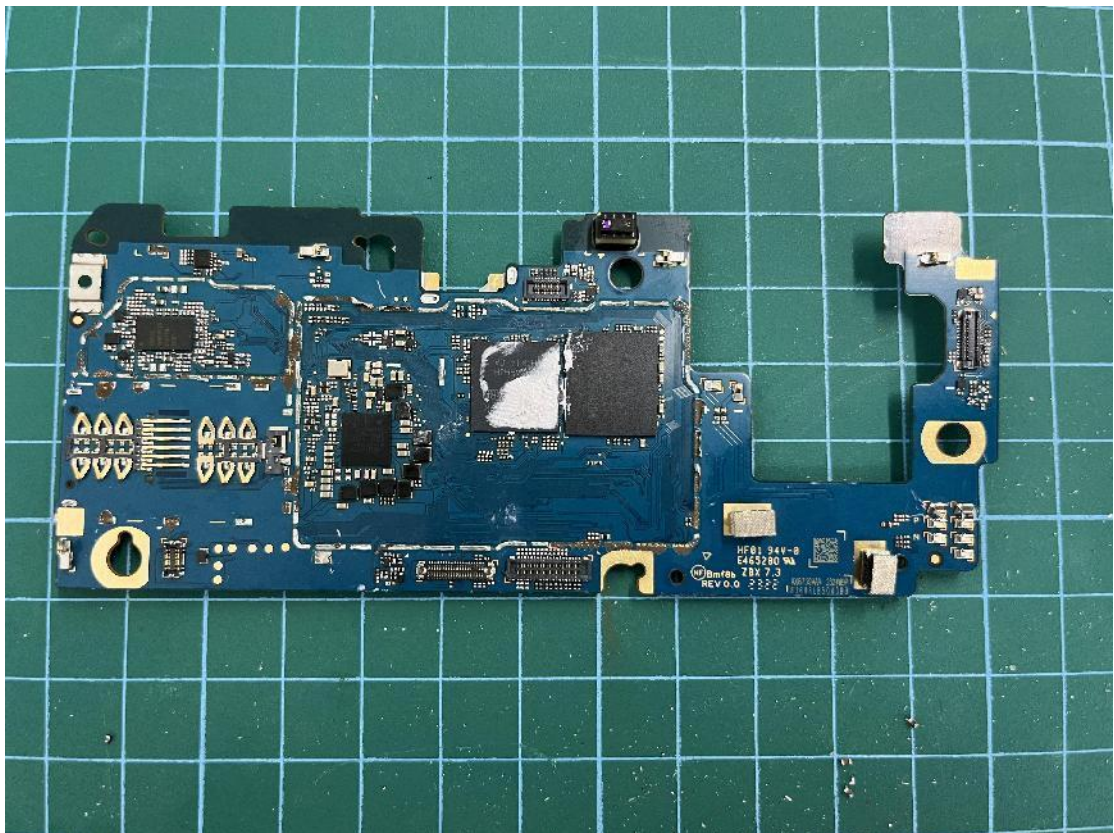
PCB10
