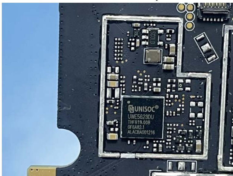
WLAN/BT/GNSS Chip
