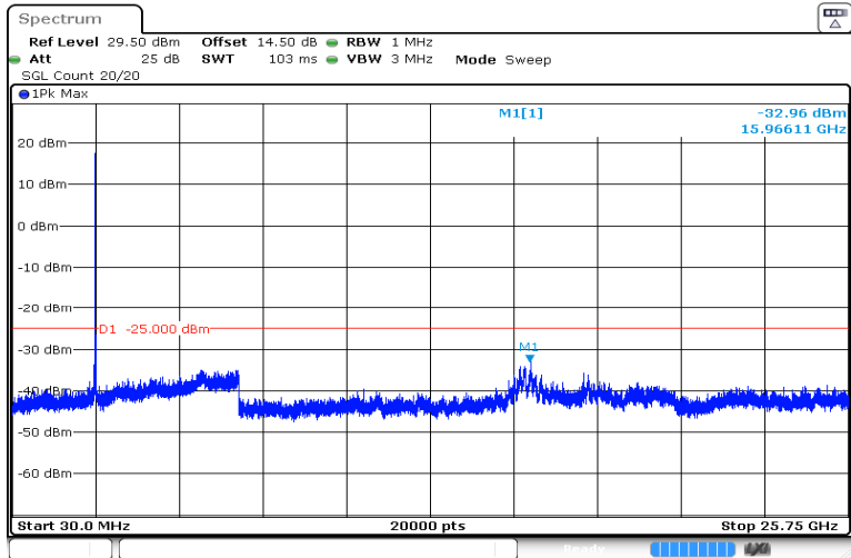
10MHz_Low_QPSK_50@0 -32.96 dBm
