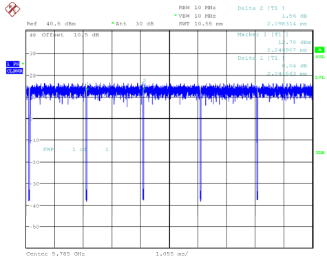
802.11a mode
