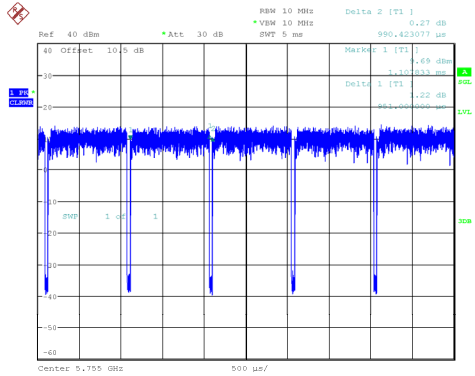
802.11ac40 mode
