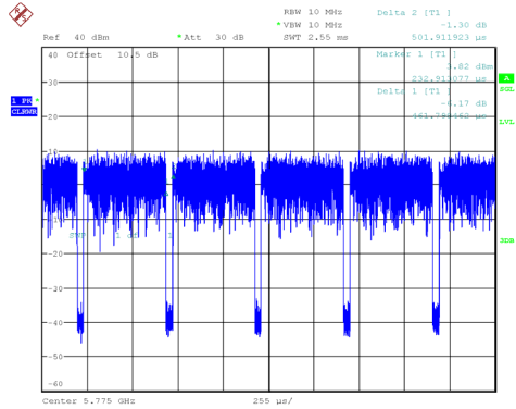
802.11ac80 mode
