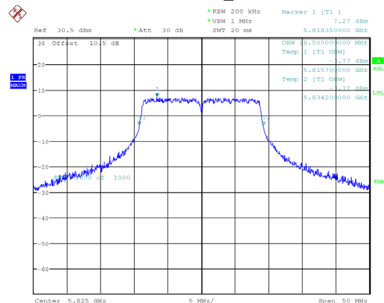
802.11ac20_5825MHz
