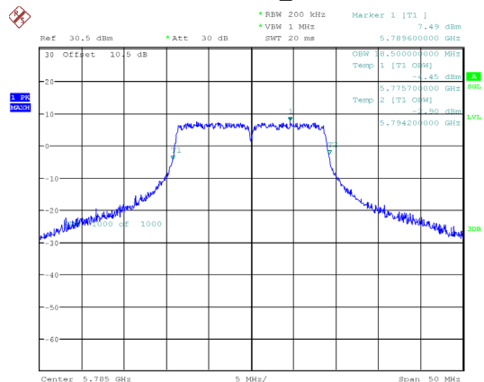
802.11ac20_5785MHz
