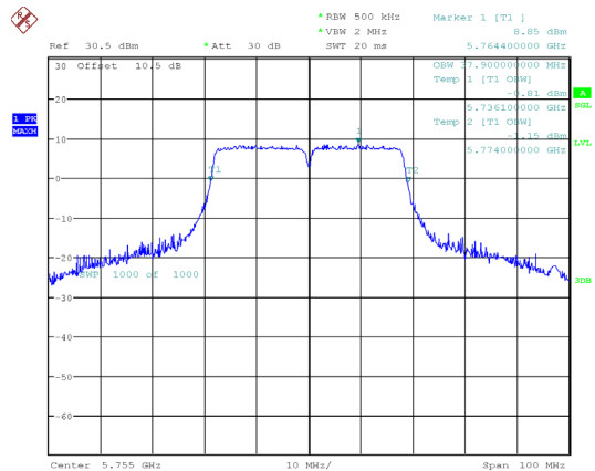
802.11ac40_5755MHz
