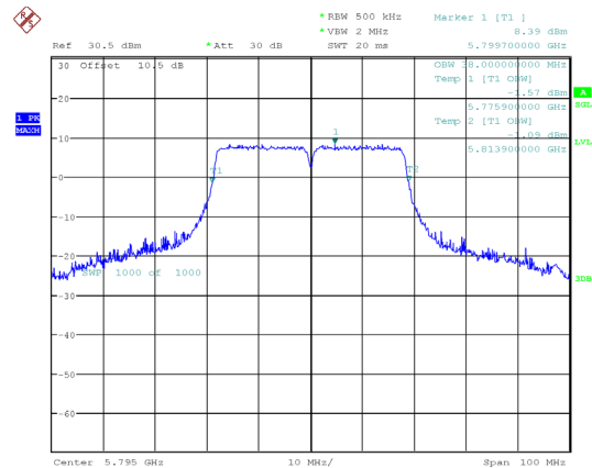
802.11ac40_5795MHz
