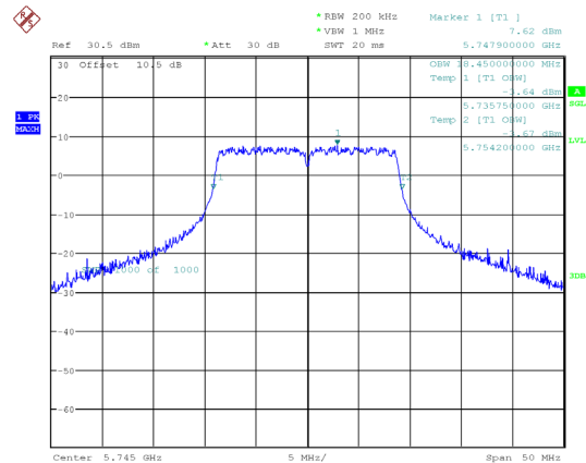
802.11ac20_5745MHz
