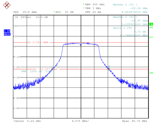
802.11ac20_5240MHz
