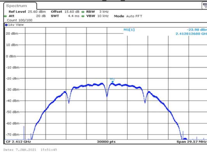
11B-CDD_Ant2_2412
