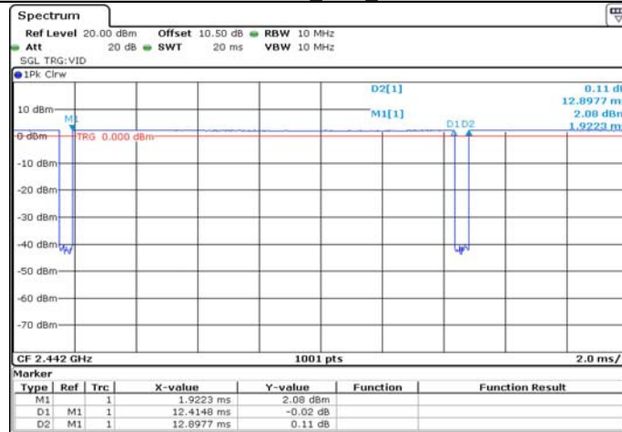
11BMIMO_Ant1_2442
