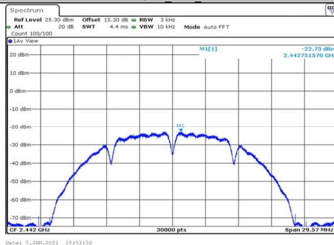
11B-CDD_Ant1_2442
