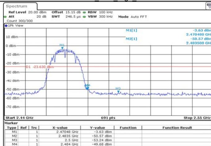
11B-CDD_Ant1_High_2472
