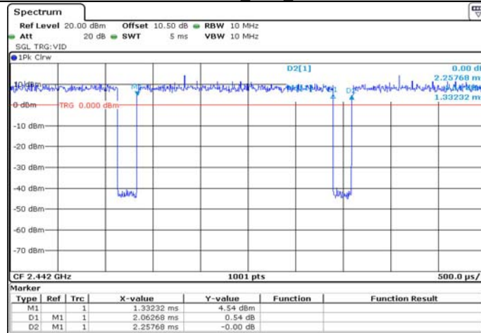
11GMIMO_Ant1_2442
