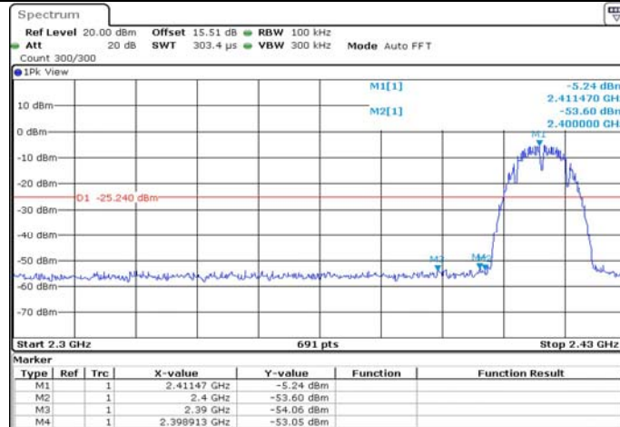
11B-CDD_Ant2_Low_2412
