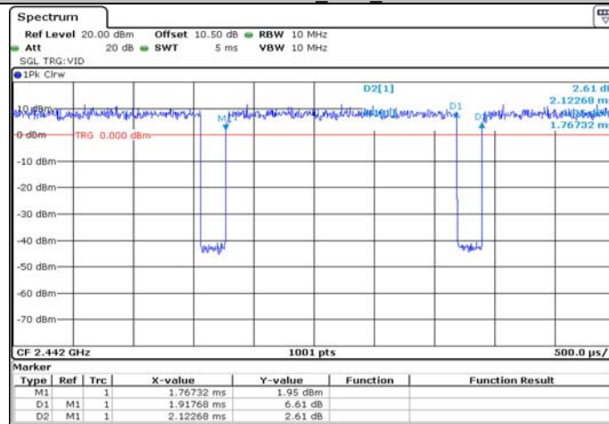
11N20MIMO_Ant1_2442
