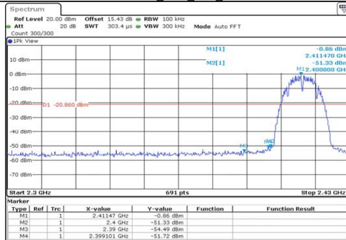
11B-CDD_Ant1_Low_2412
