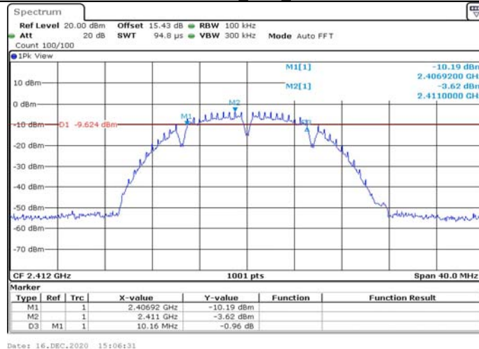
11BMIMO_Ant2_2412
