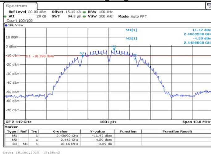
11BMIMO_Ant1_2442
