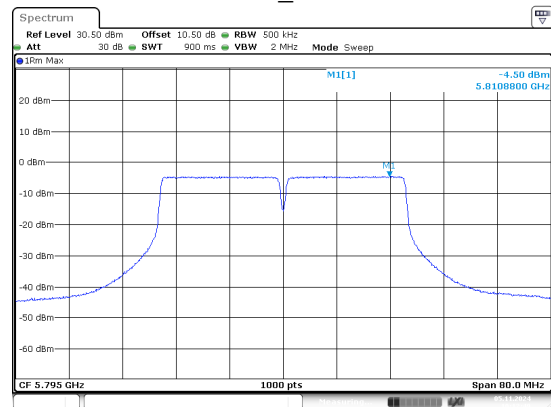
802.11n40_5795MHz
