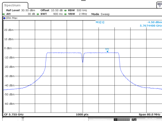
802.11n40_5755MHz
