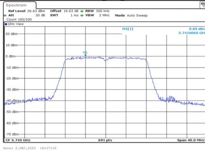
11AMIMO_Ant2_5745
