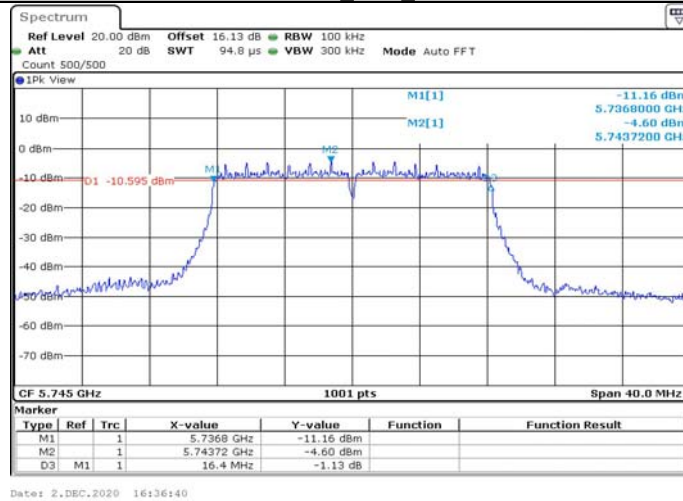
11AMIMO_Ant2_5745
