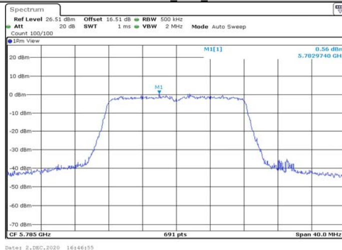
11AMIMO_Ant1_5785
