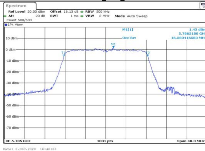
11AMIMO_Ant1_5785
