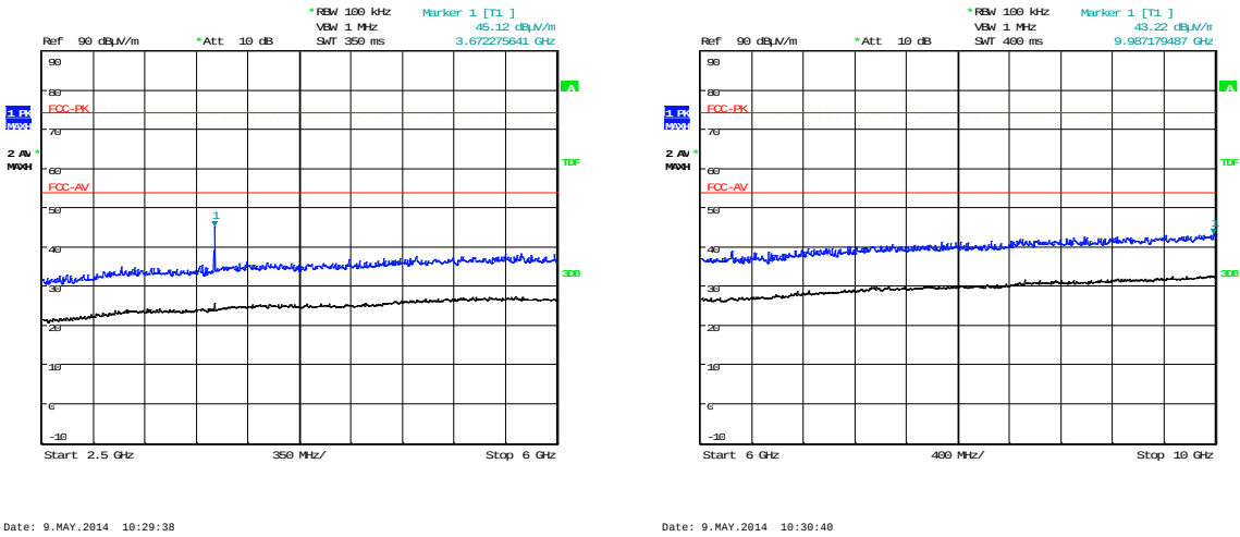
2.5GHz – 6GHz
