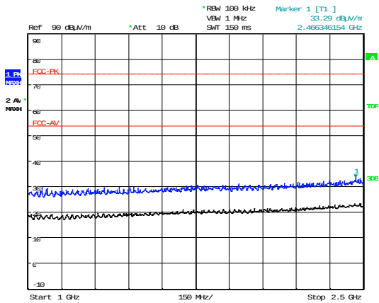
1GHz – 2.5GHz
