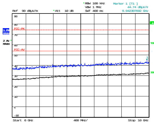
6GHz – 10GHz
