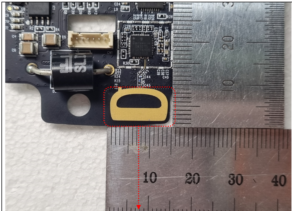
Antenna
