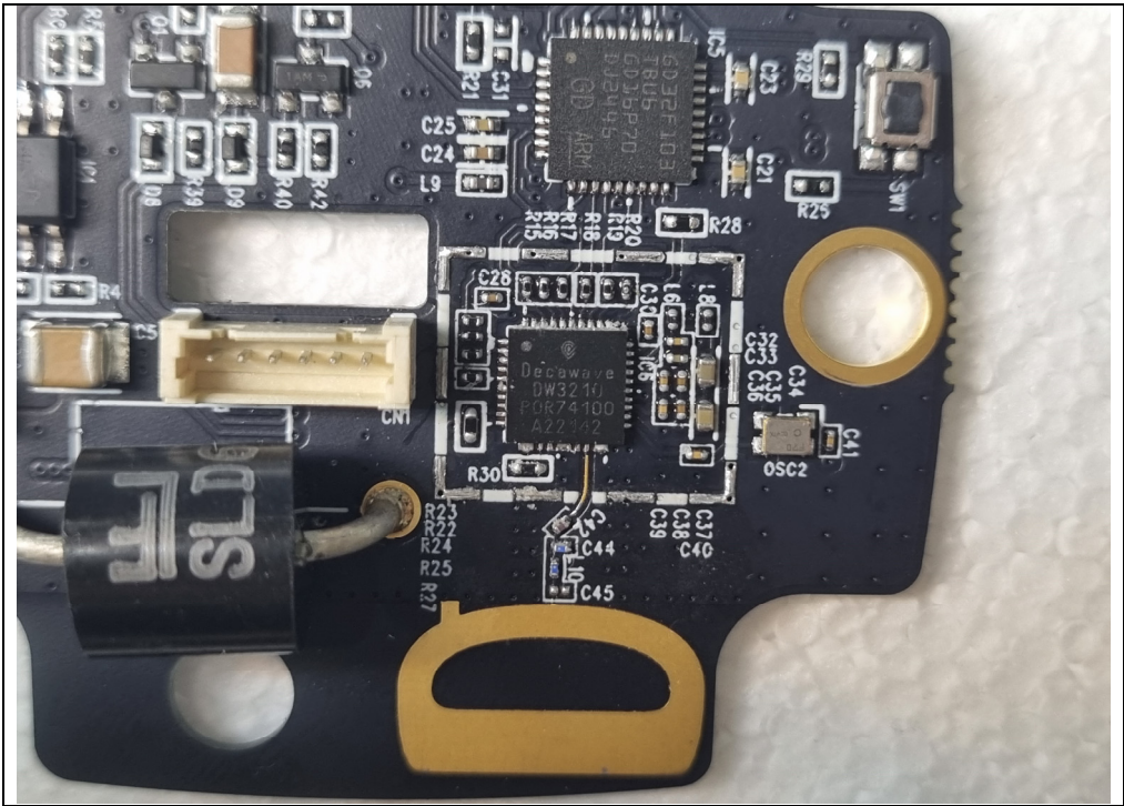
UWB part
