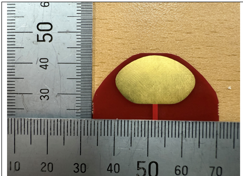
Antenna
