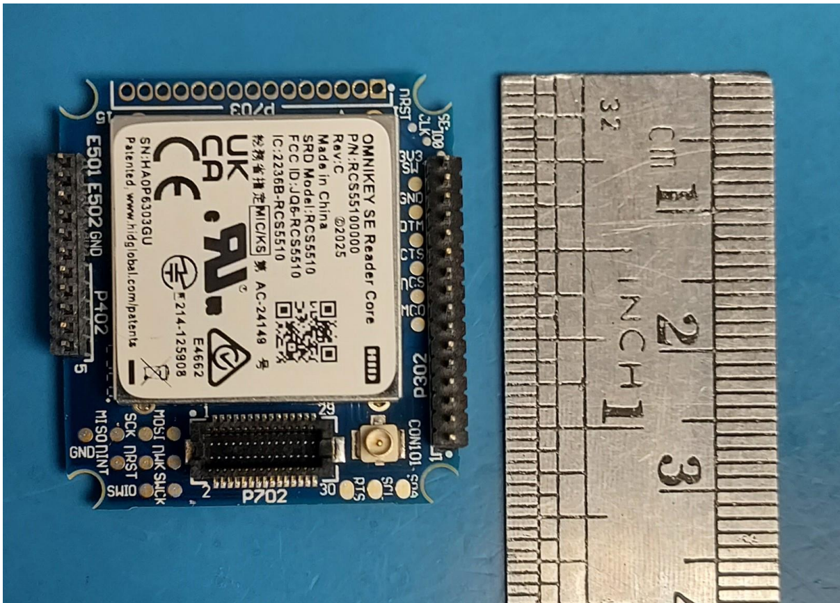
RFID module top view
