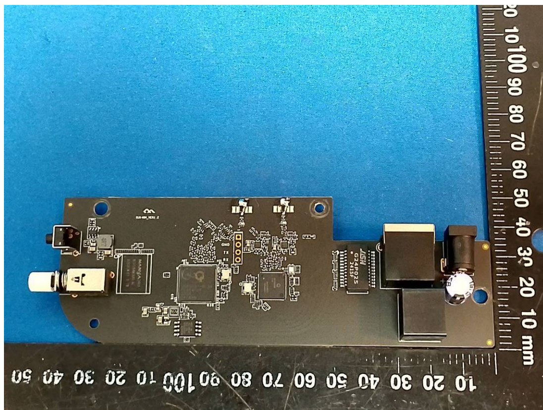
2.4G +5G module
