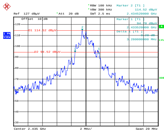
CH08, 2435MHz
