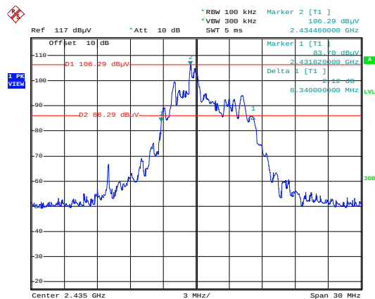
CH08, 2435MHz
