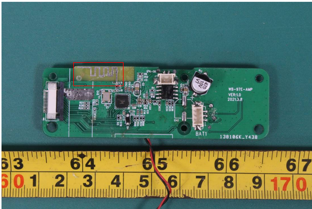
Antenna
