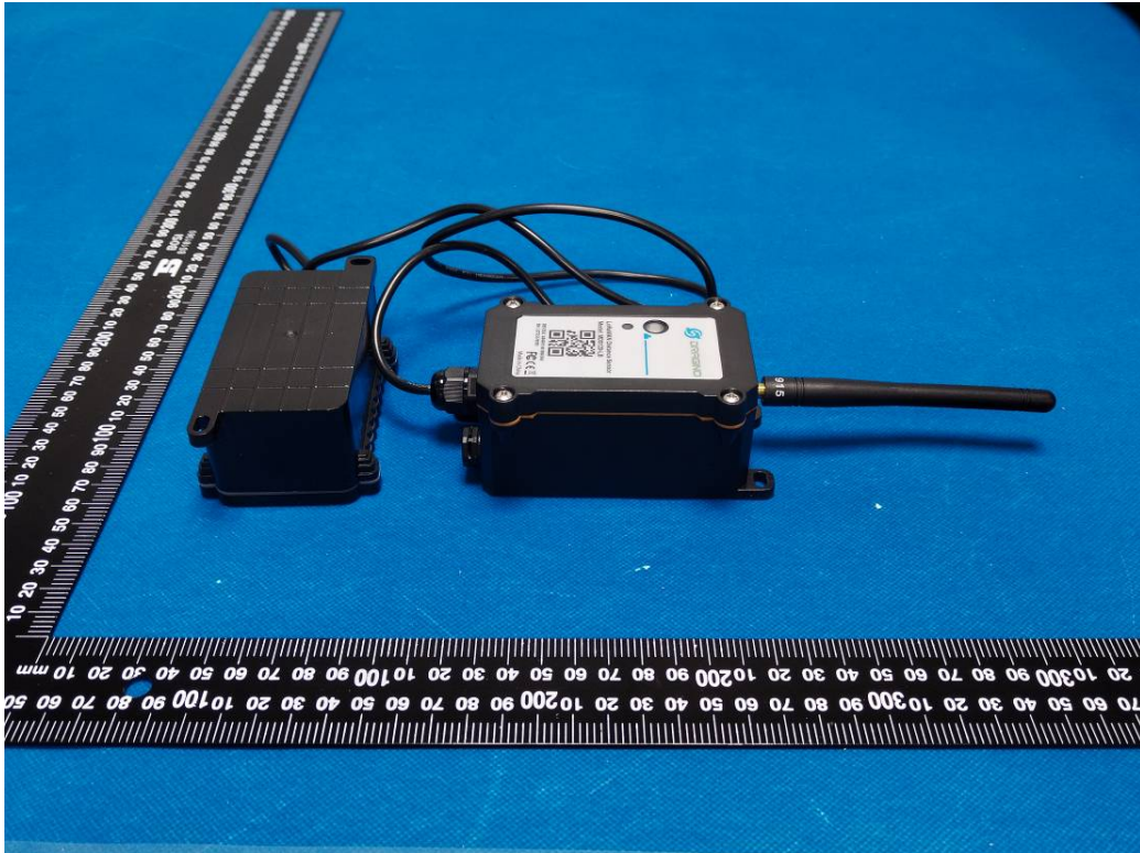
MDS200-LB
