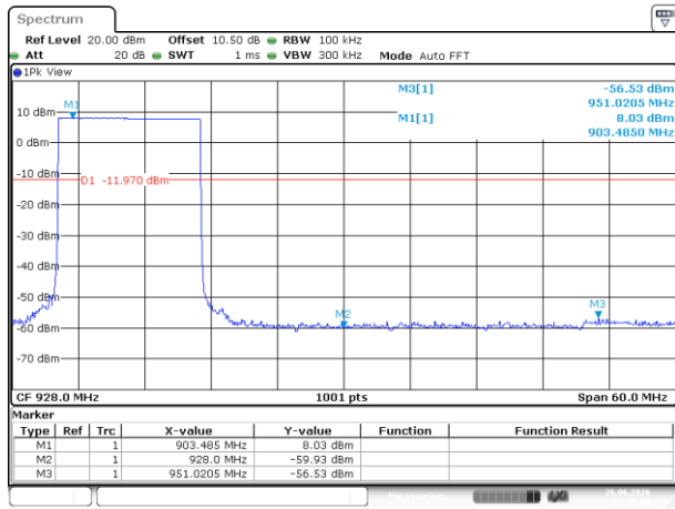
Lora 125k_Hopping_Upper
