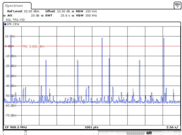
Lora 125k_Hopping
