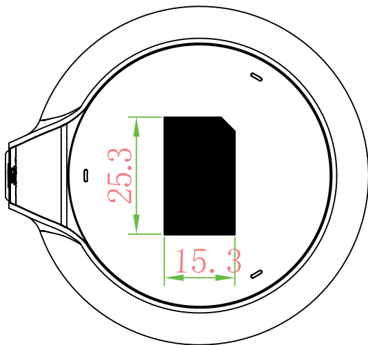
BC161 主机贴纸粘贴位置——底面预留位置
