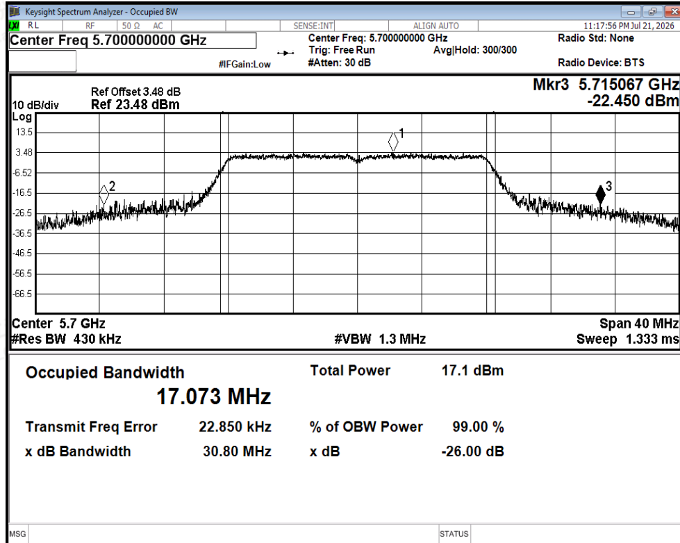
-26dB Bandwidth NVNT a 5700MHz Ant2
