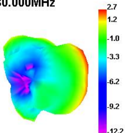
2480.000MHz
