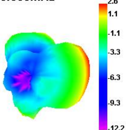
2400.000MHz
