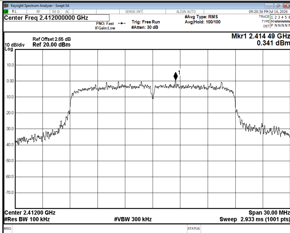
Band Edge NVNT ax20 2412MHz Ant2 Ref
