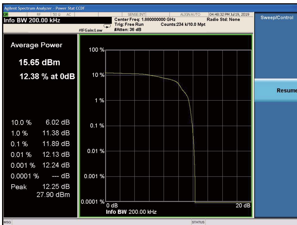
1880MHz-CH661-8PSK
