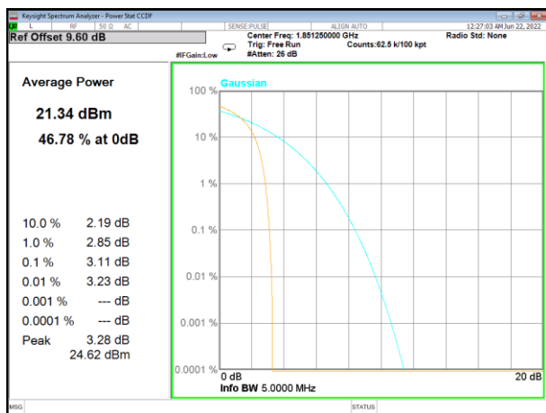
BC1_EVDO_Lower
