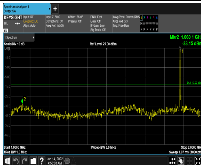
Band25-3MHz-QPSK-26365-1RB#0-Range2:1000~2000MHz
