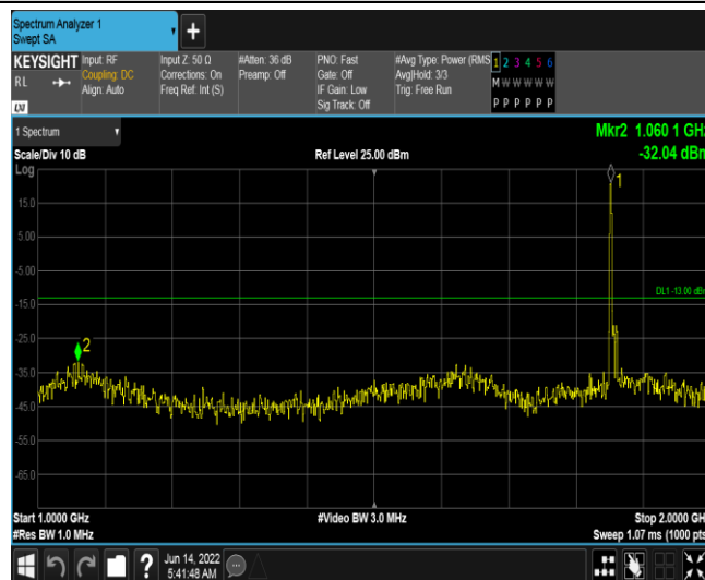
Band25-5MHz-QPSK-26065-1RB#0-Range2:1000~2000MHz
