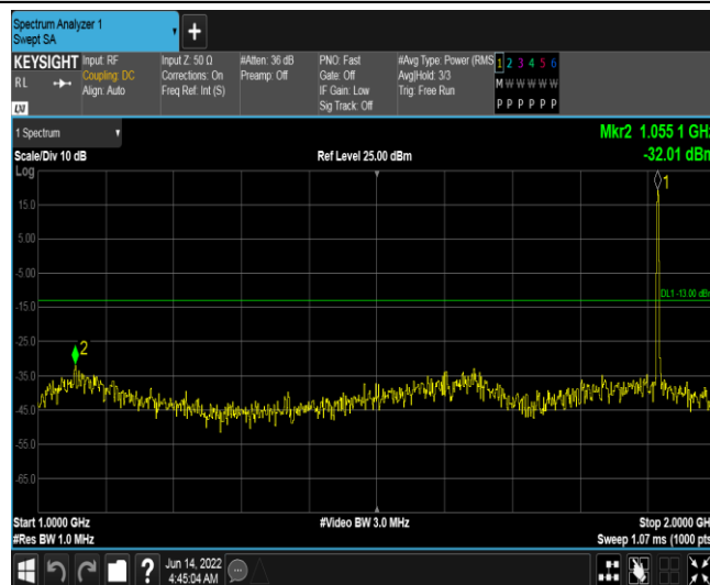
Band25-1.4MHz-QPSK-26683-1RB#0-Range2:1000~2000MHz
