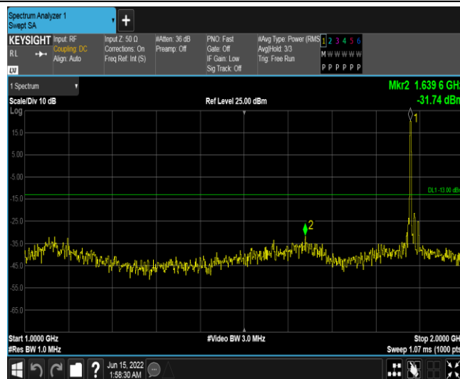
Band25-10MHz-16QAM-26365-1RB#0-Range2:1000~2000MHz
