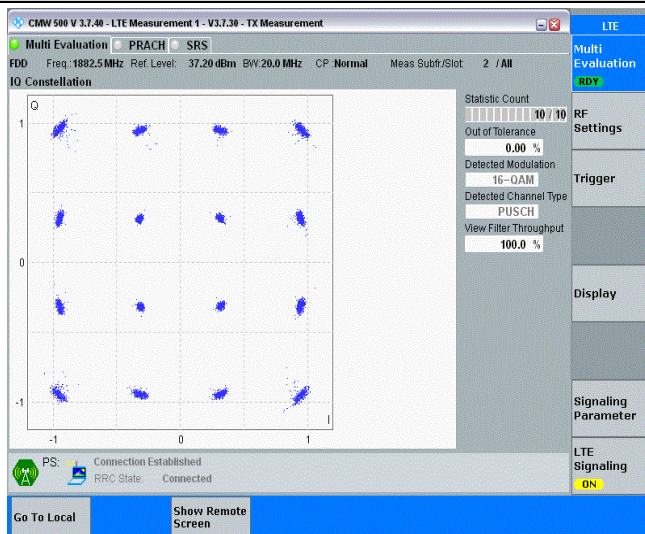
Band25-20MHz-16QAM-26365-100RB#0
