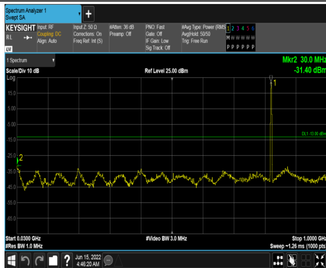
Band26-1.4MHz-QPSK-26797-1RB#0-Range2:30~1000MHz
