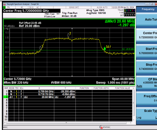
11N20MIMO Ant9 5720
