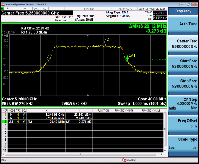
11N20MIMO Ant9 5260
