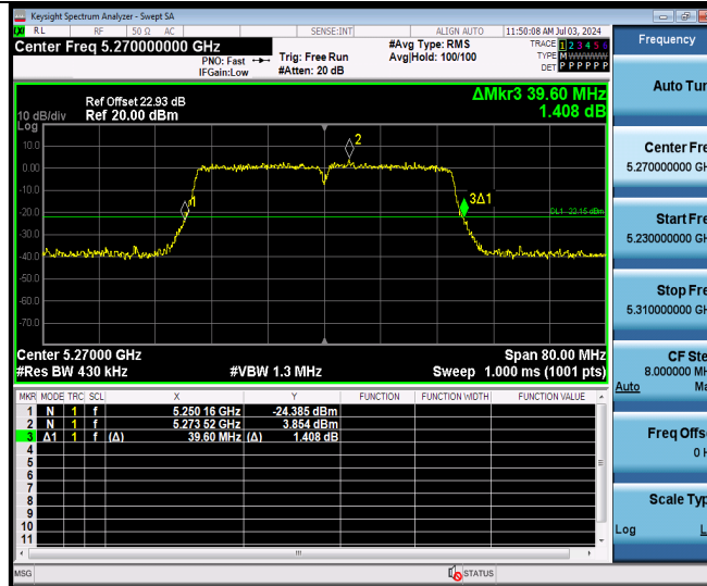
11N40MIMO Ant9 5270
