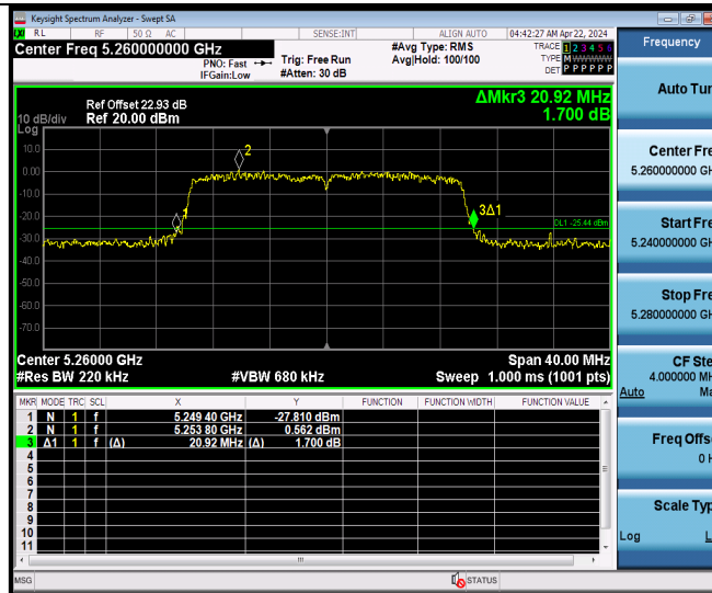
11AX20MIMO Ant9 5260
