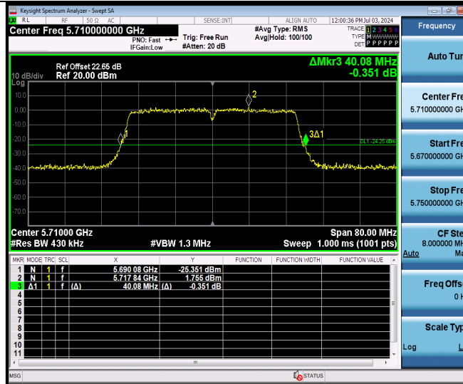
11N40MIMO Ant9 5710
