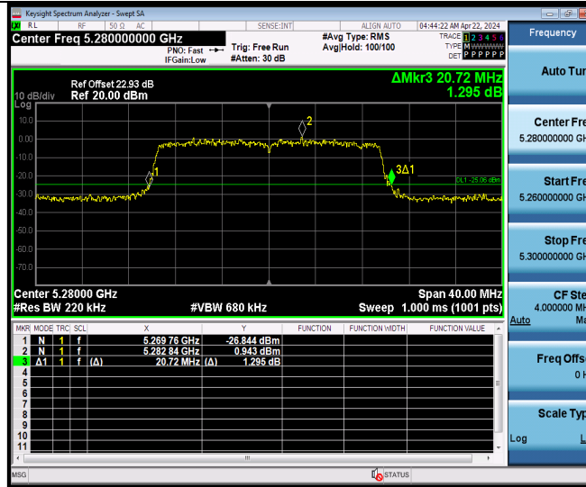
11AX20MIMO Ant9 5280
