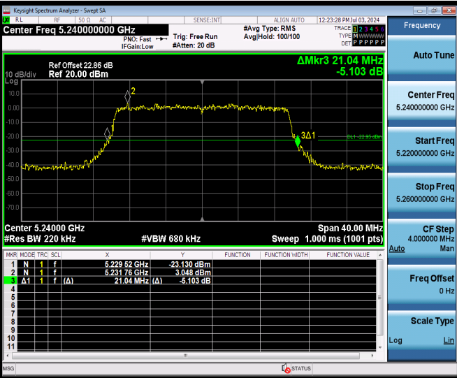
11AX20MIMO Ant9 5240
