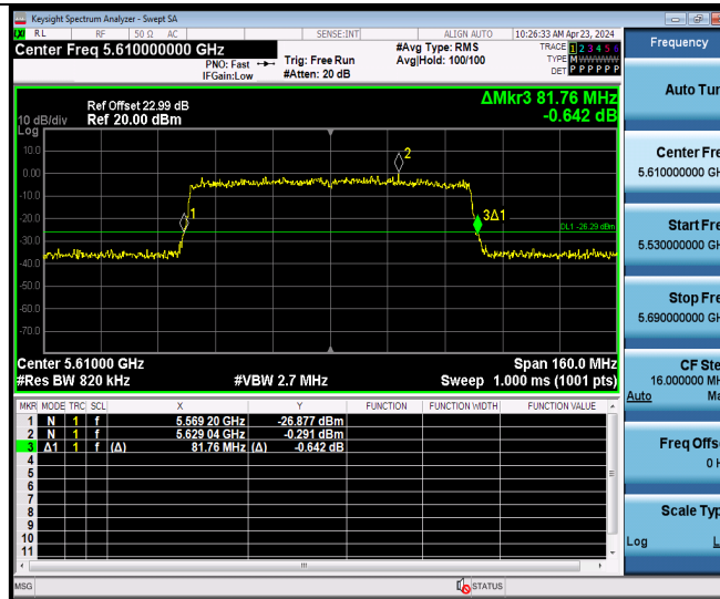
11AX80MIMO Ant9 5610
