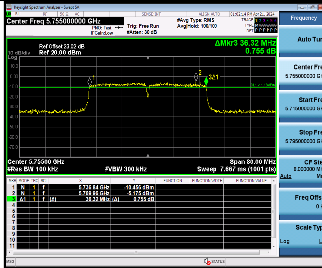
11N40MIMO Ant9 5755
