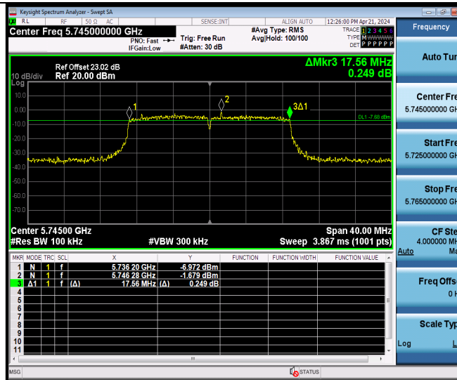
11N20MIMO Ant9 5745
