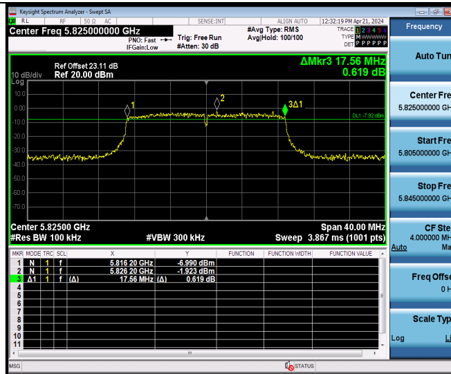
11N20MIMO Ant9 5825
