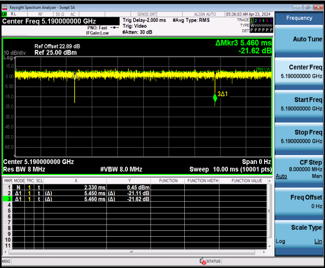
11AX40MIMO Ant9 5190
