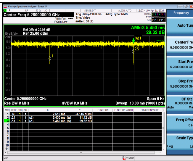
11N20MIMO Ant9 5260
