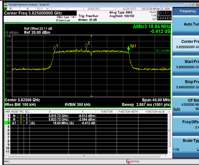
11AX20MIMO Ant9 5825
