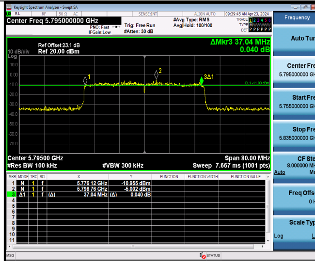
11AX40MIMO Ant9 5795
