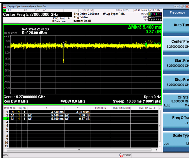
11AX40MIMO Ant9 5270
