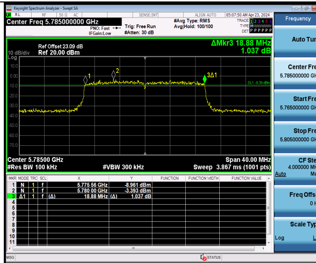
11AX20MIMO Ant9 5785
