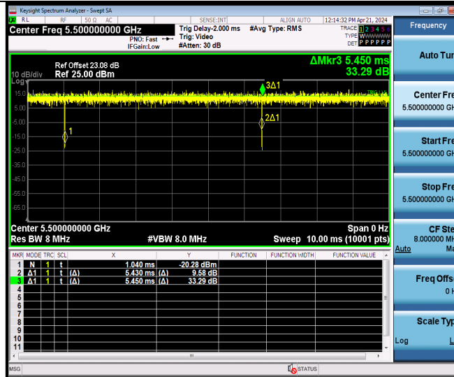
11N20MIMO Ant9 5500
