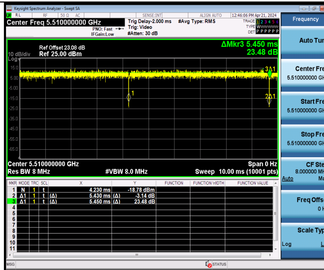
11N40MIMO Ant9 5510
