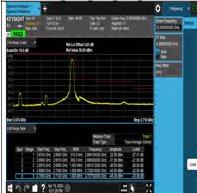
Band41 15MHz QPSK 41515 1RB#74
