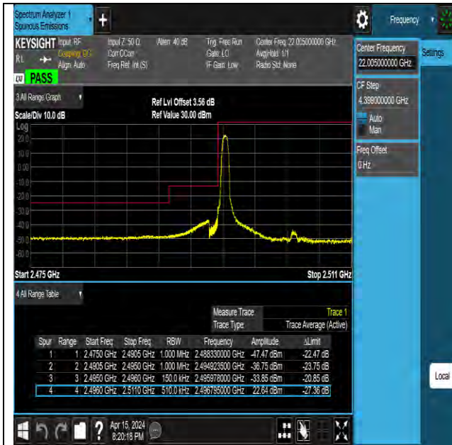
Band41 15MHz QPSK 39725 1RB#0
