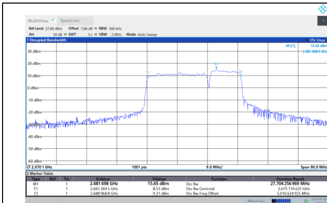
41-41-20MHz-10MHz-64QAM-64QAM-40571-40715-1 00RB#0-50RB#0
