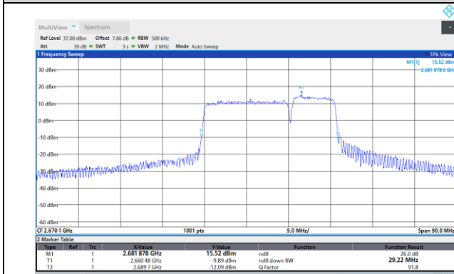
41-41-20MHz-10MHz-64QAM-64QAM-40571-40715-1 00RB#0-50RB#0
