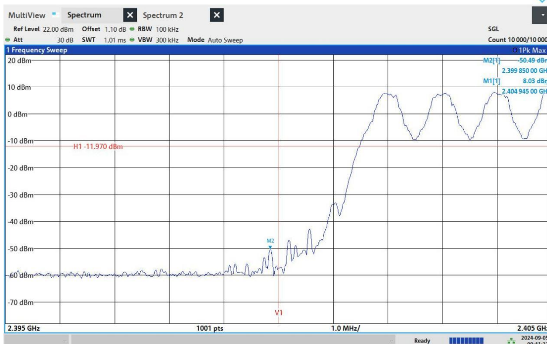
DH5_ANT0_Low_Hop_2402
