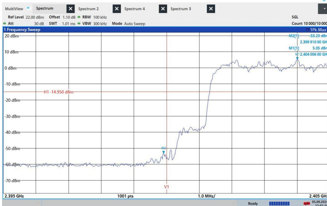
3DH5_ANT0_Low_Hop_2402
