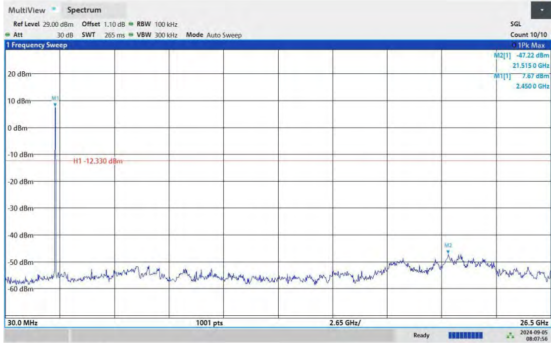
11G_Ant0_2412_30~265000
