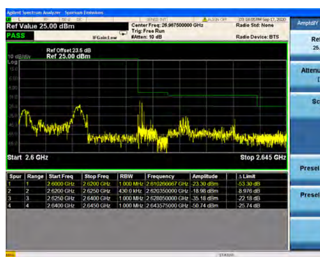
Band38 / 20MHz / High CH / QPSK / 1 RB
