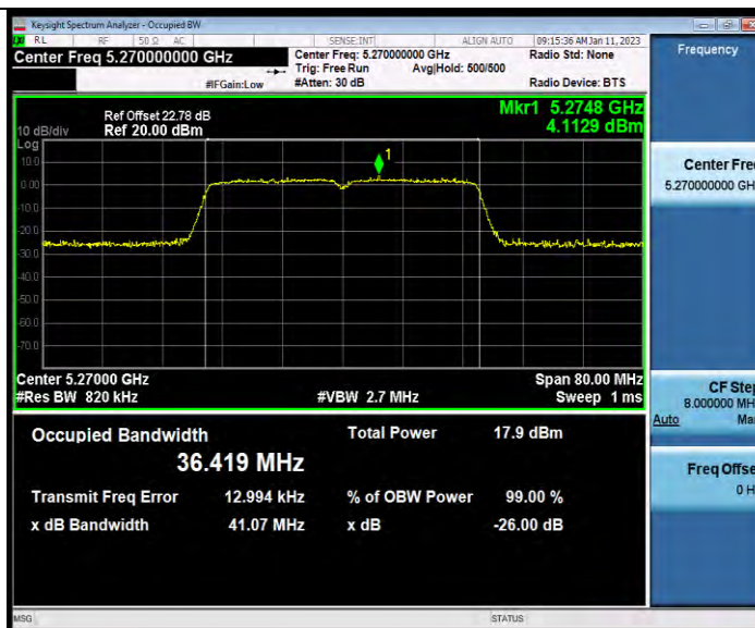
11AC40MIMO_Ant2_5270
