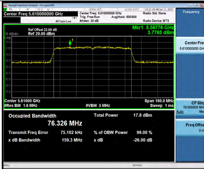
11AC80MIMO_Ant2_5610
