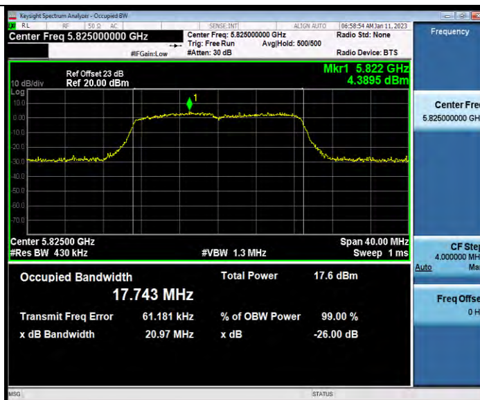
11AC20MIMO_Ant2_5825
