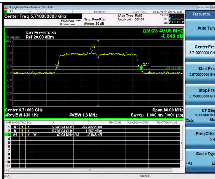
11N40MIMO_Ant2_5710
