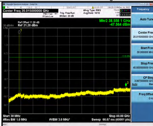
Band42-5MHz-QPSK-43065-1RB#0-Range1:30~40000MHz
