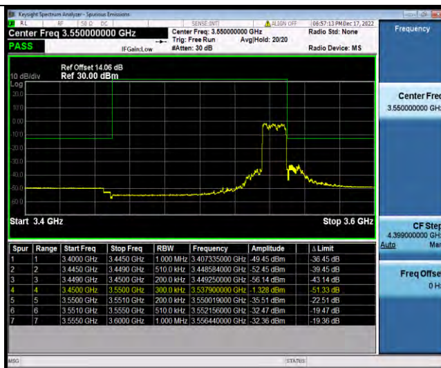
Band42-20MHz-QPSK-42190-1RB#0
