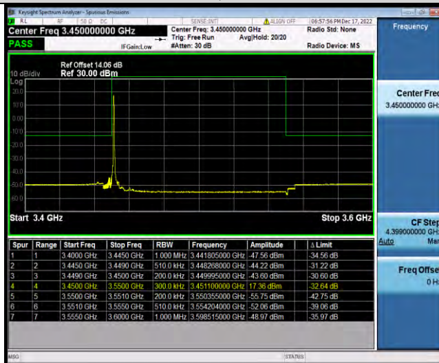
Band42-20MHz-QPSK-42190-100RB#0
