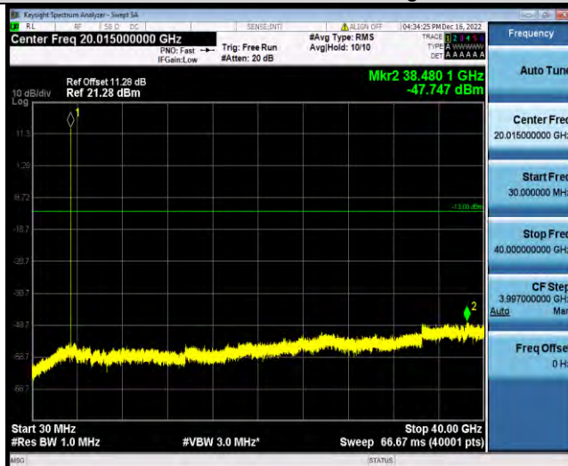
Band42-5MHz-QPSK-42590-1RB#0-Range1:30~40000MHz
