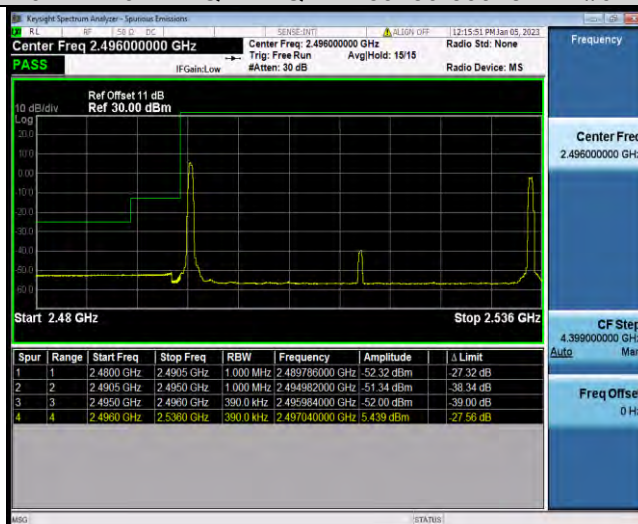
41-41-20MHz-20MHz-QPSK-QPSK-39750-39948-1RB#99-1RB#0
