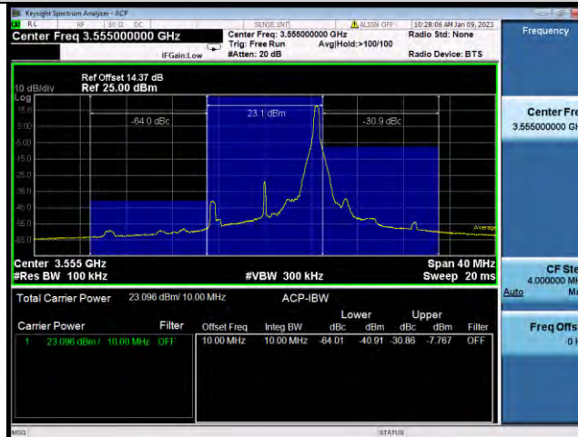
N48-10MHz-QPSK-637000-25RB#0
