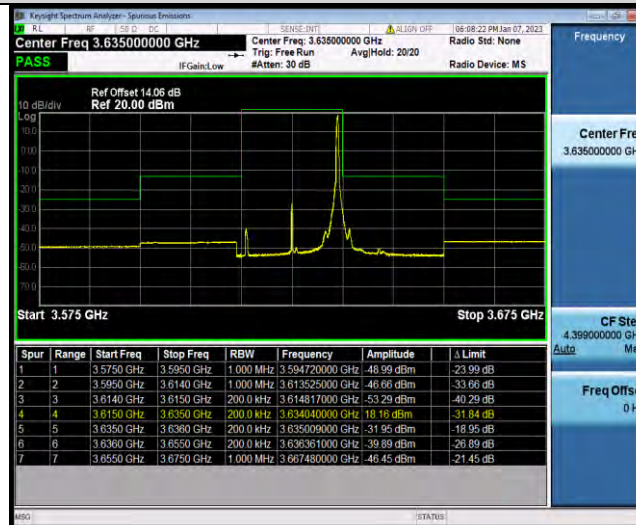
N48-20MHz-QPSK-641666-50RB#0
