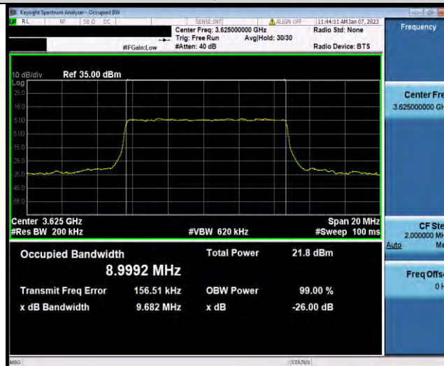
N48-10MHz-64QAM-641666-25RB#0
