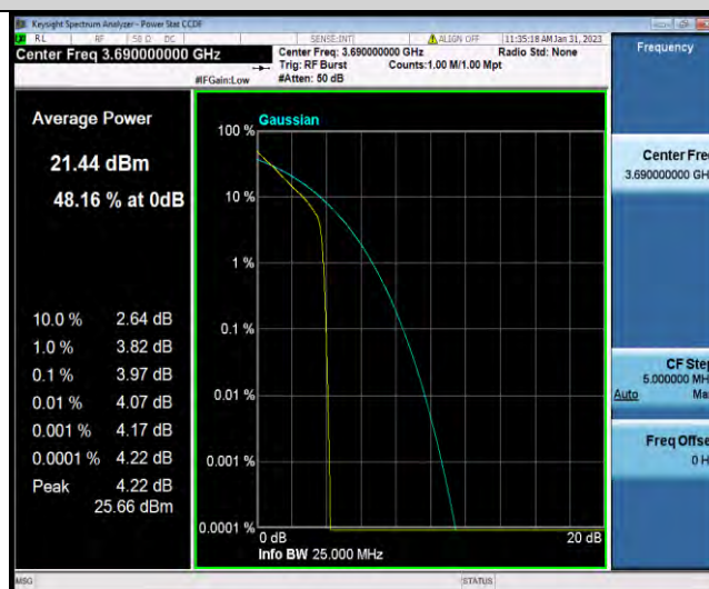
N48-20MHz-QPSK-646000-50RB#0
