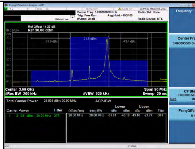
N48-20MHz-QPSK-646000-50RB#0
