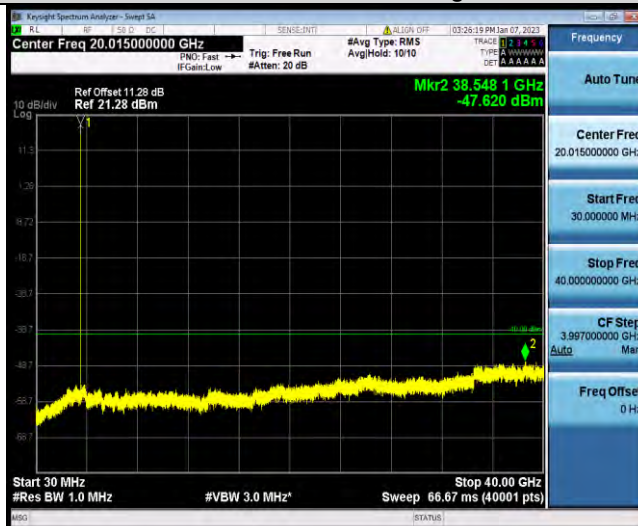
N48-10MHz-QPSK-641666-1RB#0-Range1:30~40000MHz
