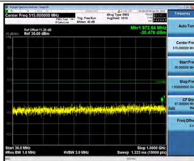
N25-5MHz-QPSK-376500-1RB#0-Range1:30~1000MHz
