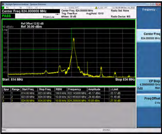
N5-5MHz-QPSK-165300-25RB#0
