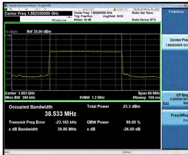
N25-40MHz-BPSK-376500-216RB#0
